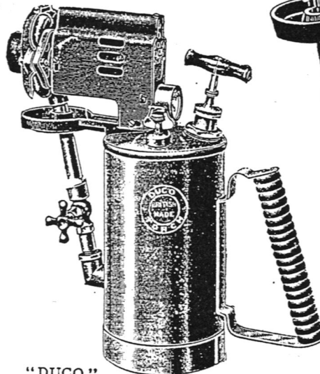
„DUCO“ (Barthel System). British made.
